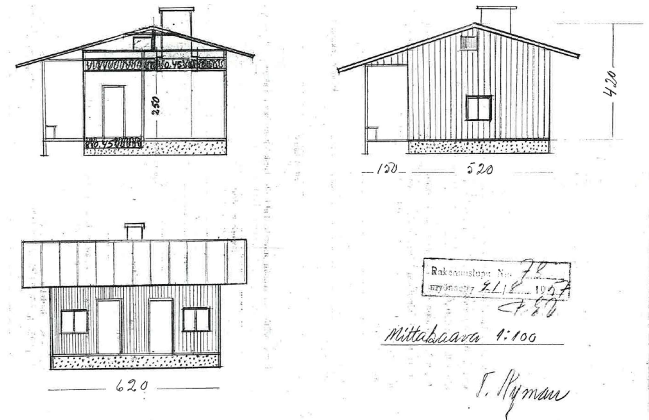
Kuva 7. Kiinteistön länsiosassa olevan saunarakennuksen (nykyinen ranta-aitta) rakennuslupapiirustukset vuodelta 1957.
