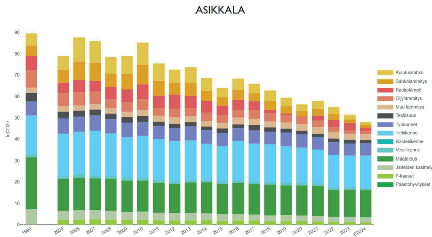
Kuvaaja 1. Asikkalan kunnan alueella syntyneiden ilmastopäästöjen kehitys vuosien 2005-2024 välillä. (Lähde: Syke – Kuntien ja alueiden khk-päästöt, hiilineutraalisuomi.fi)
